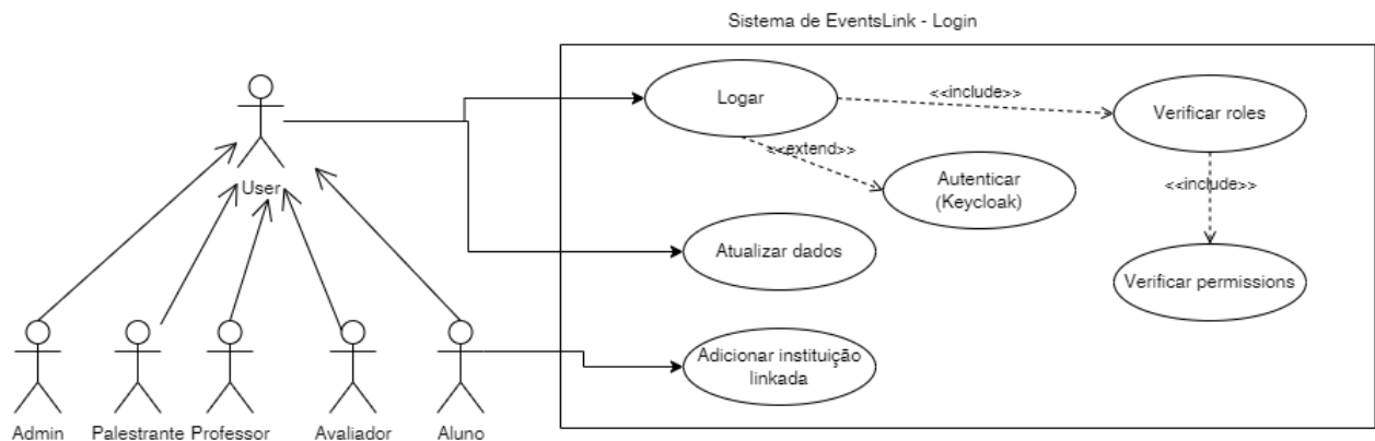
Figura 23 - Diagrama de Caso de uso Login
