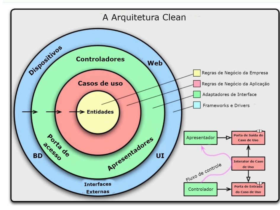
Figura 3 - Arquitetura Clean
