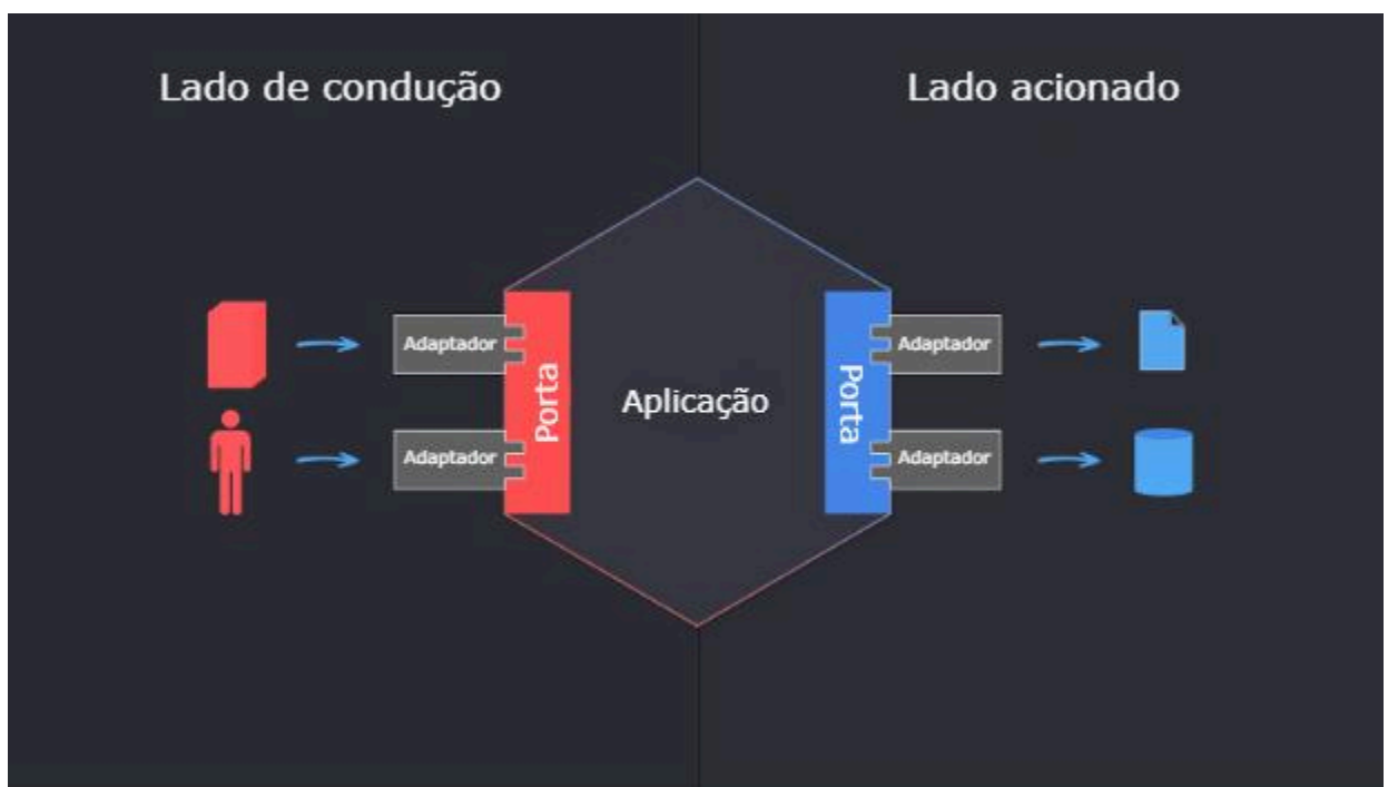
Figura 4 - Arquitetura Hexagonal
