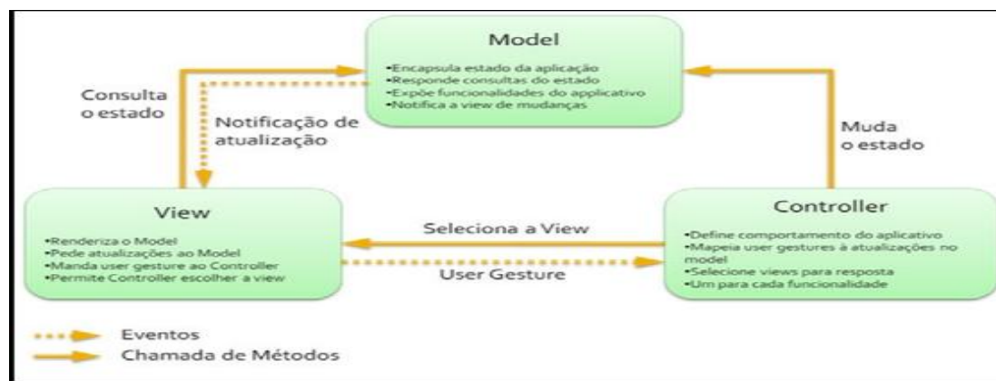
Figura 5 - Arquitetura MVC
