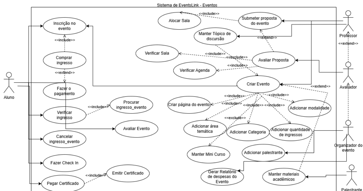
Figura 25 - Diagrama de Caso de uso Eventos
